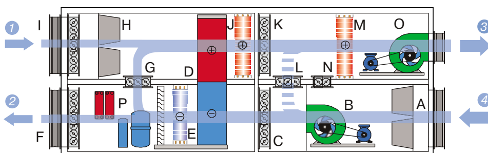
Модель Х (пластинчатый рекуператор)
