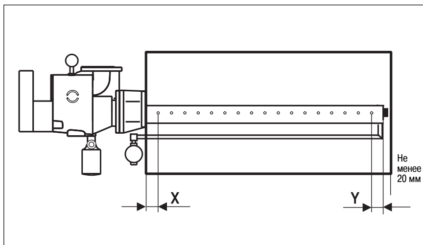
Размеры блока с несколькими раздающими патрубками
