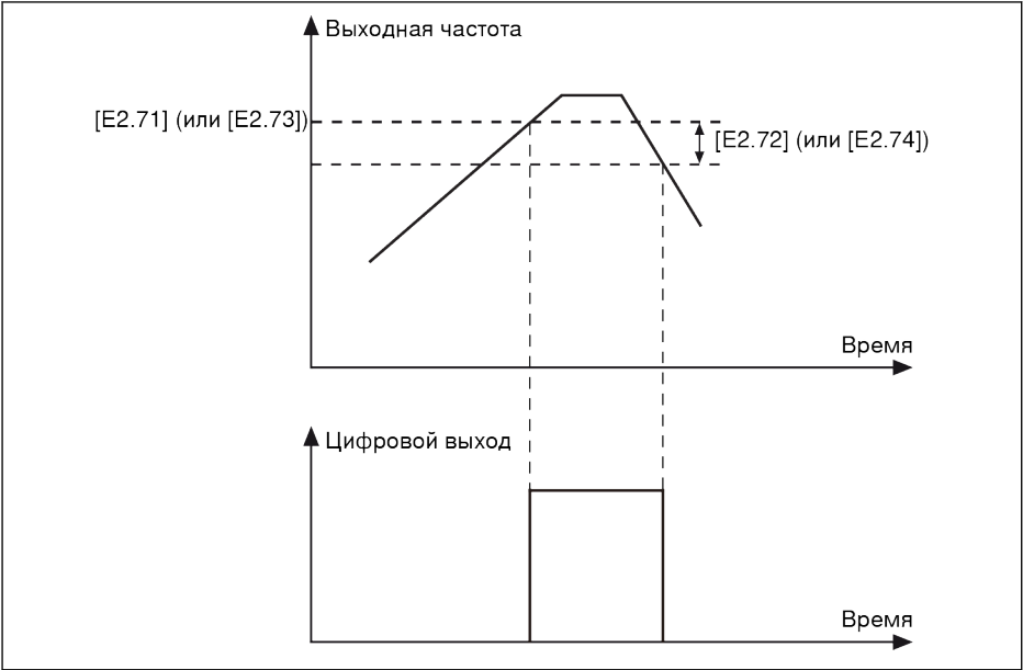
Рис. 12-41: Обнаружение уровня частоты
