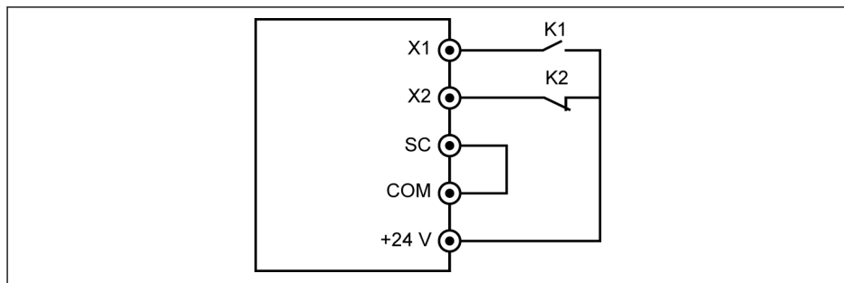
Рис. 12-53: Сигнал ошибки
