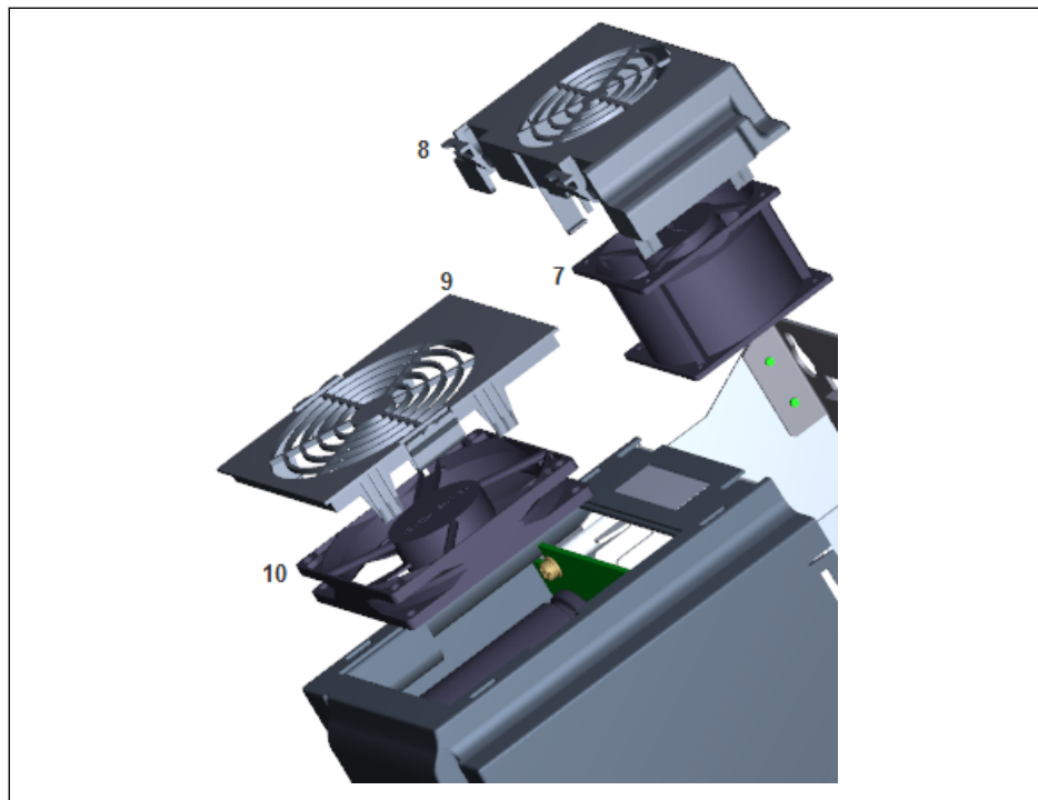
Рис. 16-3: Разборка вентилятора
