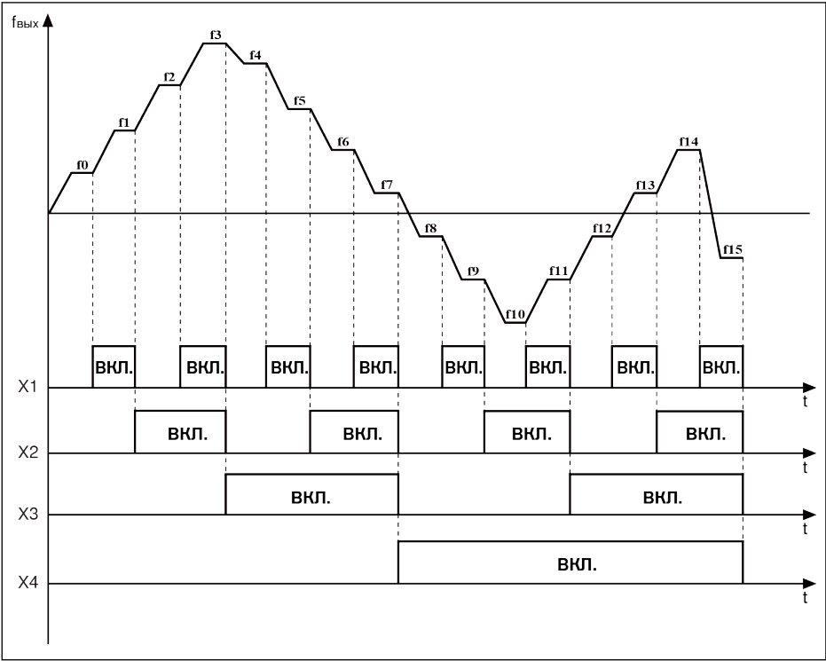
Рис. 12-17: Переход в фазу многоскоростного режима
