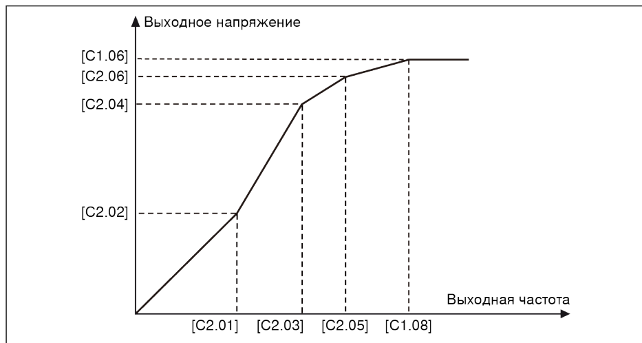
Рис. 12-62: Задаваемая пользователем кривая V/f при [C2.05] \leq [C1.08]
