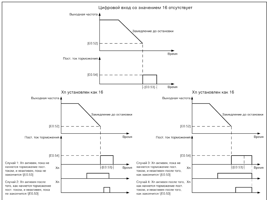
Рис. 12-29: Остановка торможения пост. током
